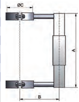
Rohrschlitten Zoll pipe holder slide-type inch
