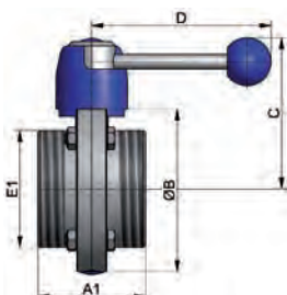
butterfly valve SV04 inch MM handle HB04 item-no. 55504-
