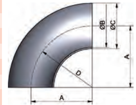
Schweißbogen DIN 11852-BS 90° CC welding bend DIN 11852-BS 90° CC
