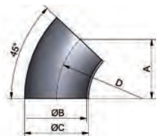
Schweißbogen DIN 11852-BS 45° CC welding bend DIN 11852-BS 45° CC
