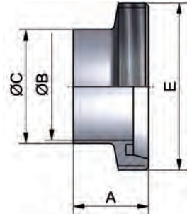
Kegelstutzen Zoll welding liner inch
