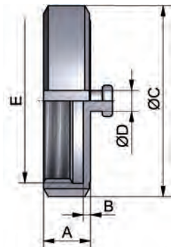
Blindmutter (komplett)
