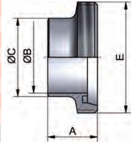
Kegelstutzen SD welding liner
