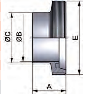
Kegelstutzen DIN 11851-SD
